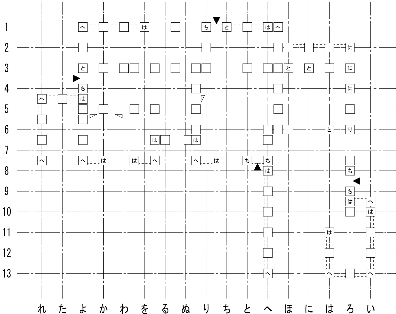
1階柱壁伏図
